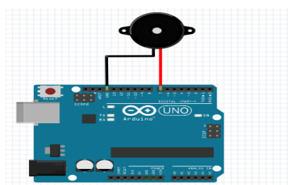
Gambar 4: Perancangan arduino UNO dengan buzzer
