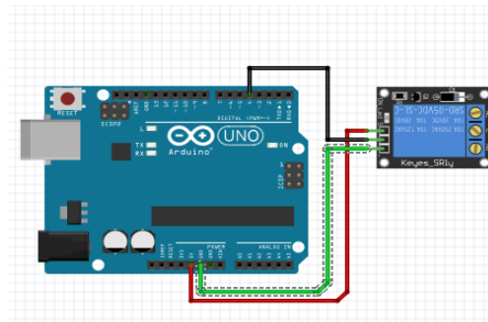
Gambar 3 : Perancangan arduino UNO dengan Relay
