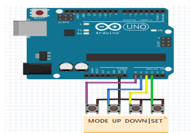
Gambar 5: Perancangan arduino UNO dengan Push Button
